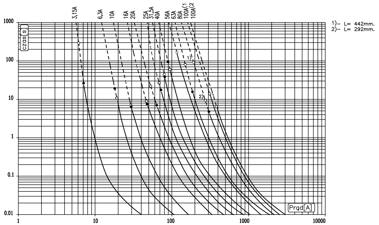
Rys. 2 Charakterystyki czasowo-prądowe wkładek typu BMW-7,2/3,15–100A (bez 63 A 0 I = 292 mm); BMW-12/3,15–40A oraz 63A i 80A.
