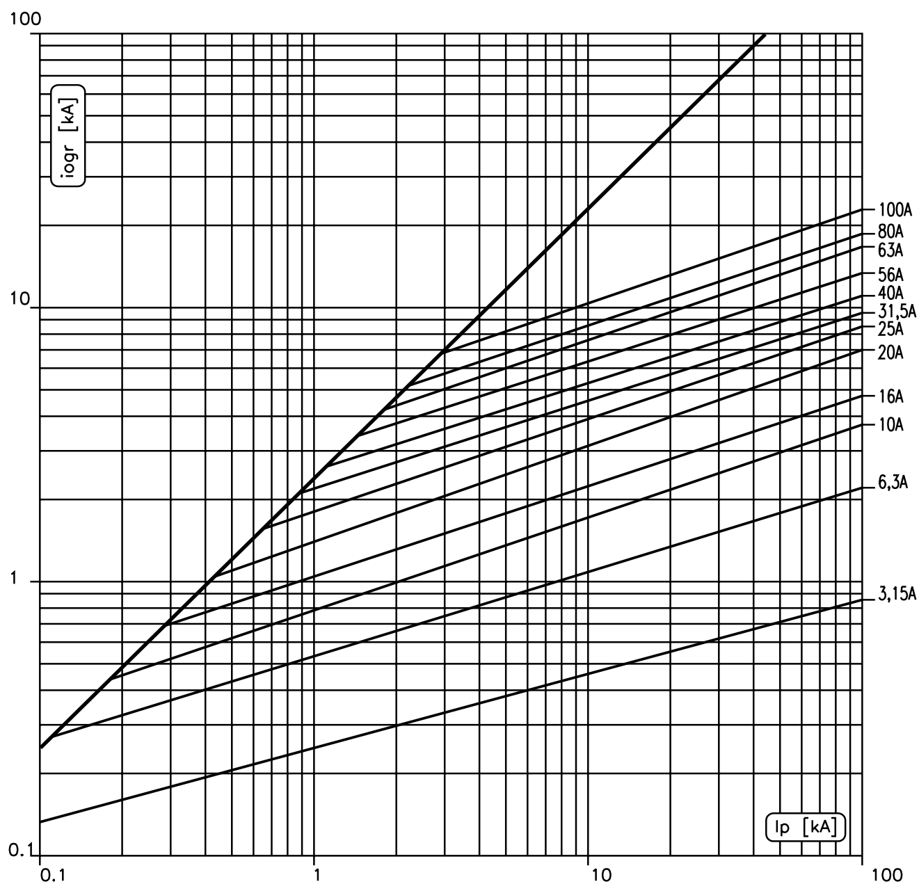
Rys. 1 Charakterystyki prądów ograniczonych wkładek bezpiecznikowych typu BMW–7,2; 12; 24; 36 kV.
