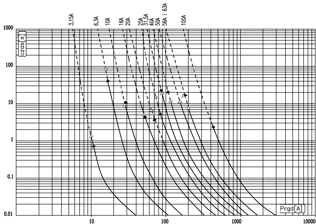
Rys. 3 Charakterystyki czasowo-prądowe wkładek typu BMW-7,2/63A (wymiar L = 292\text{ mm} ); BMW-24/3,15–63A; BMW-12/56 i 100A oraz BMW-36/3,15–40A
