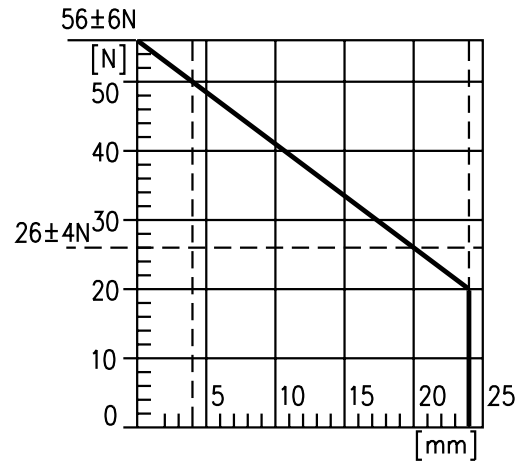
Charakterystyka wybijaka F-L.
